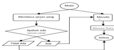
Gambar 10. Diagram Aktivitas Komunikasi Kotak Pesan Oleh Dosen Dan Mahasiswa
