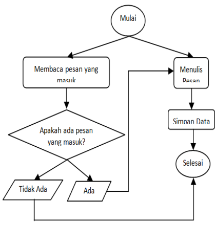
Gambar 11. Diagram Aktivitas Komunikasi Kotak Pesan
