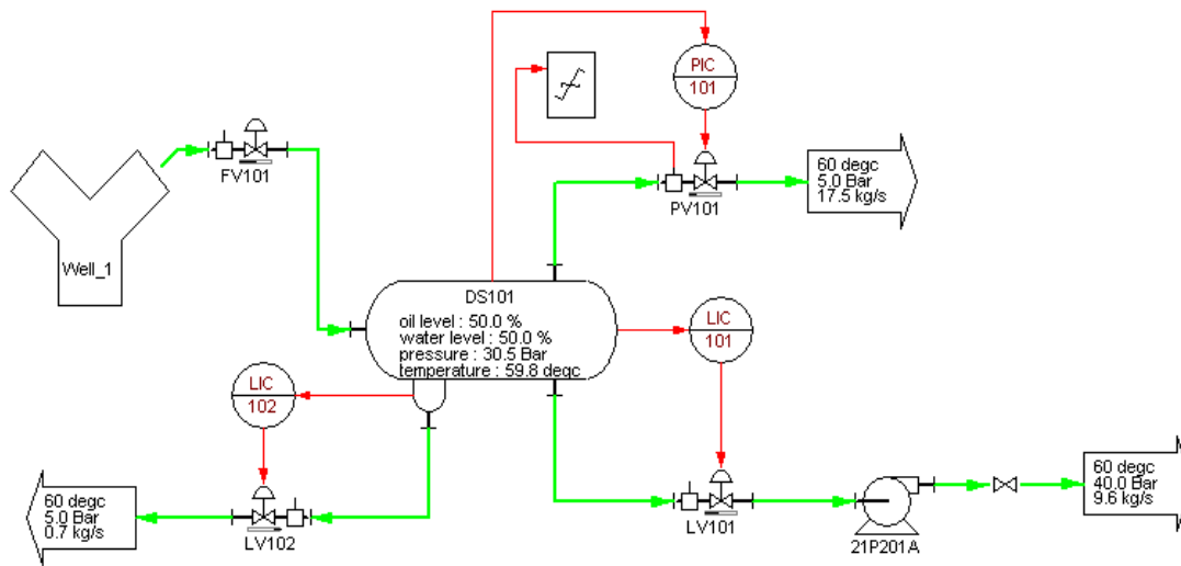
Gambar 1. Instalasi Sumur gas bumi
