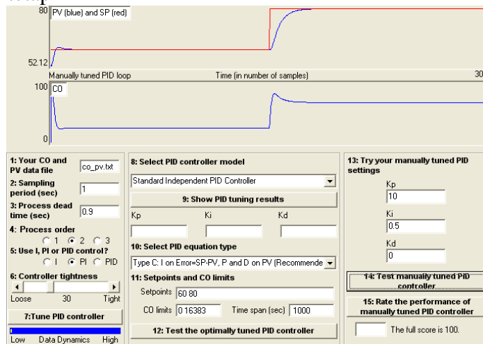
Gambar 4. Grafik Pengendali Proporsional (P) dan Integral (I)
