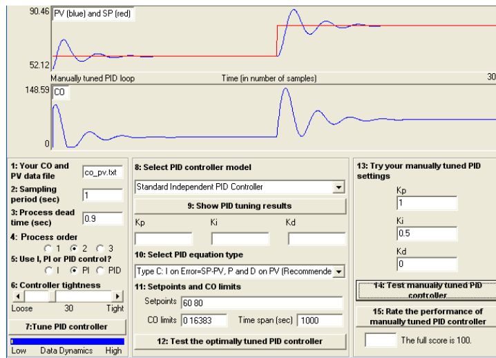
Gambar 3. Grafik Pengendali Proporsional (P) dan Integral (I)
