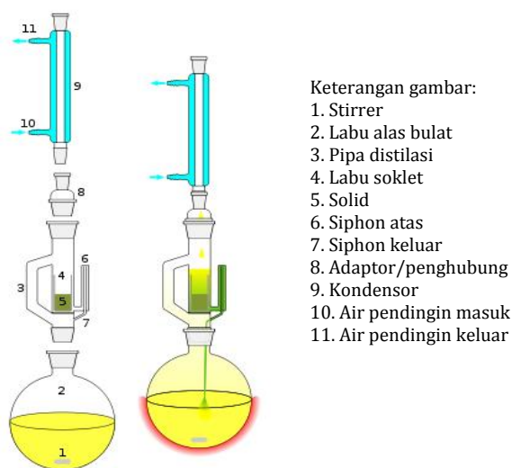
Gambar 2. Alat Ekstraksi
