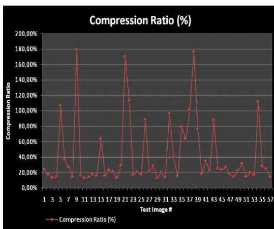
Gambar 8. Rasio kompresi dari 57 citra 24-bit BMP.
