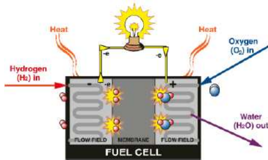
Gbr. 1. Ilustrasi prinsip kerja sel bahan bakar
