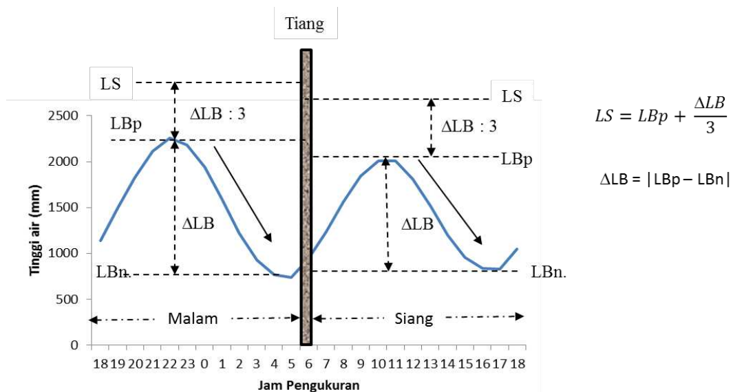
Gambar 2. Ilustrasi pengukuran tunggang air pasang surut dengan MSS.
