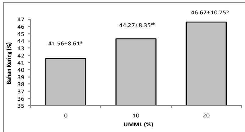
Gambar 2. Degradasi bahan kering (%) sistem rumen in vitro pakan campuran jerami padi dan tepung daun murbei dengan imbang 70:30 dan ditambahkan urea mineral molases liquid (UMML)
