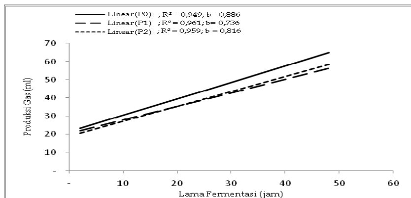
Gambar 1. Laju produksi gas hasil fermentasi ransum jerami padi dan tepung daun murbei dengan imbang 70:30
