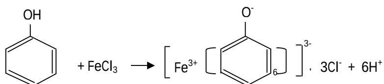
Gambar 2. Persamaan reaksi antara gugus fenol dengan \text{FeCl}_3
