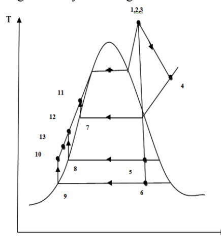
Gambar 7. Diagram T-s Sistem Pembangkit Kogenerasi
