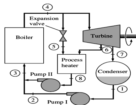
Gambar 3. Skema Sistem Pembangkit[2]
