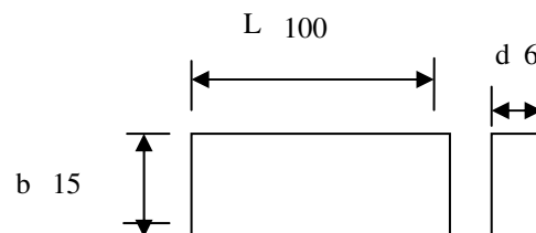
Gambar 1. Geometri dan Dimensi Spesimen Uji Bending ASTM D 790
