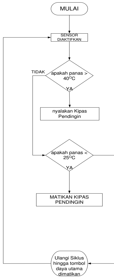
Gbr. 6. Bagan alir filosofi pengatur panas
