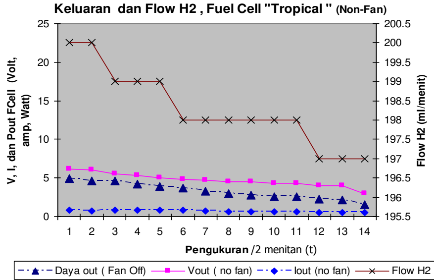
Gbr. 13a Output FC tanpa fan
