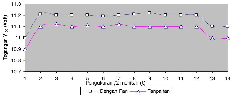
Gbr. 11. Tegangan FC tanpa beban dengan dan tanpa fan
