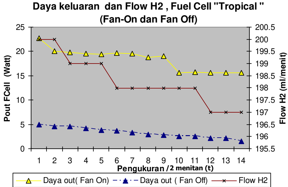
Gbr. 14. Daya keluaran FC berbeban dengan dan tanpa fan
