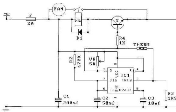
Gbr. 7. Rangkaian pengatur panas
