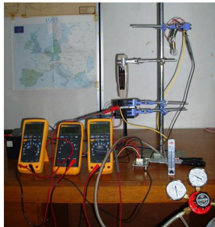
Gbr. 17. Rangkaian pengujian
