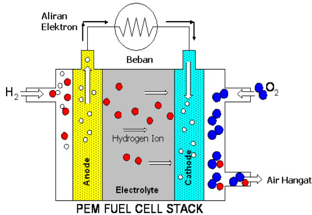
Gbr. 2. Prinsip kerja PEM FC
