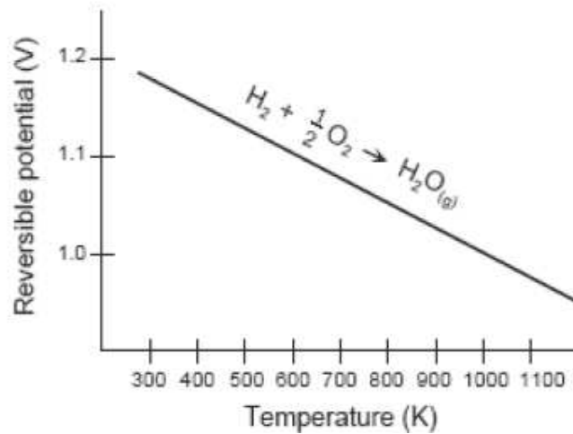
Gbr. 5. Hubungan antara temperatur dan tegangan FC (sumber: figure 2-1, FC handbook edisi 5)
