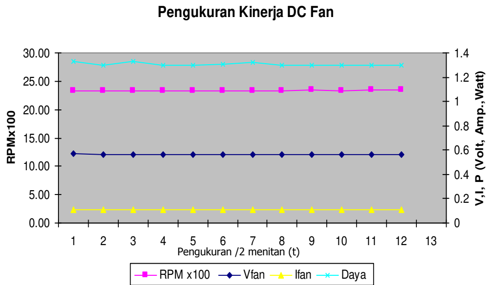
Gbr. 12. Pengukuran daya konsumsi oleh fan
