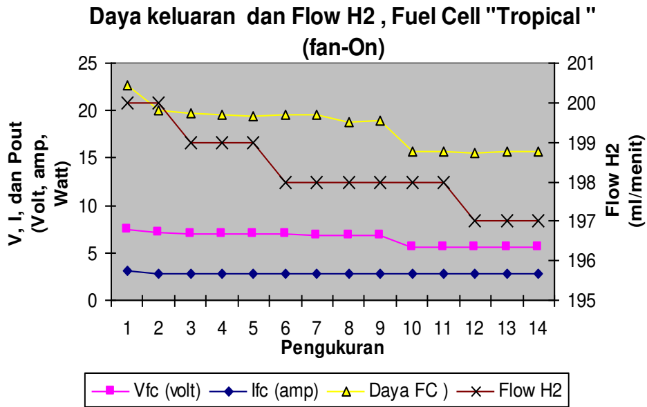
Gbr. 13b. Output Ddengan fan-
