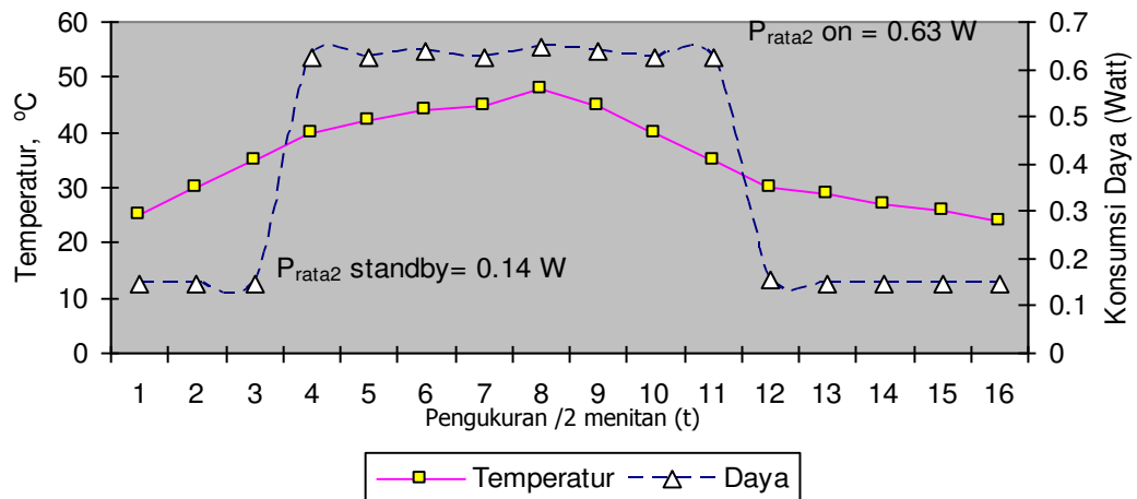
Gbr. 10. Daya konsumsi maximum dan minimum dari pengatur temperatur
