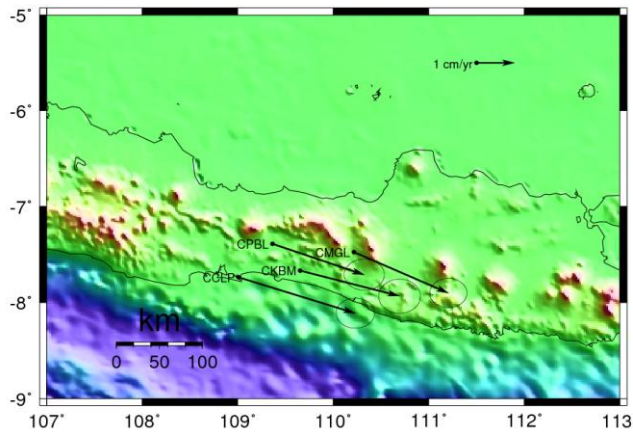
Gambar IV.4. Kecepatan pergeseran ( velocity rate ) horizontal sebelum gempa
