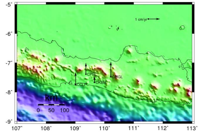
Gambar IV.7. Kecepatan pergeseran ( velocity rate ) horizontal setelah gempa
