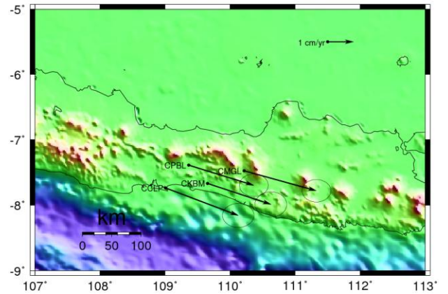
Gambar IV.5. Kecepatan pergeseran ( velocity rate ) horizontal setelah gempa
