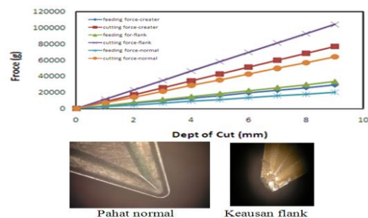
Gambar 1 Kondisi gaya potong dan gaya makan pada berbagai kondisi pahat
