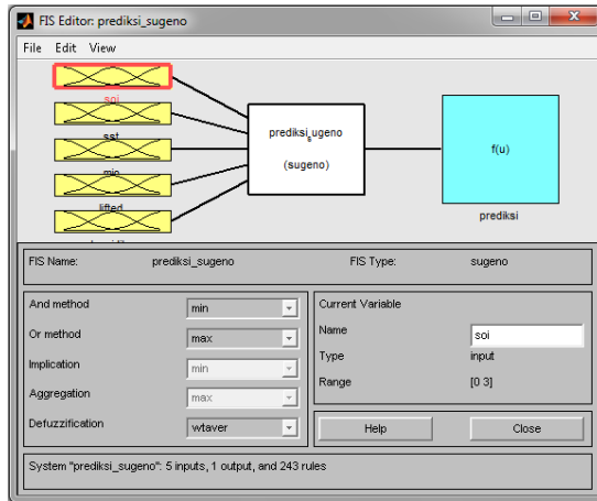
Gambar 11. FIS Editor tipe Sugeno
