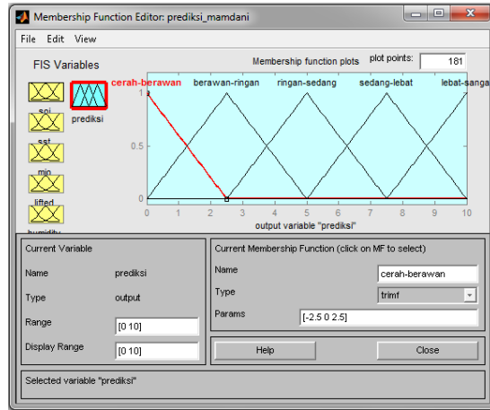
Gambar 8. MF output (prediksi) tipe Mamdani
