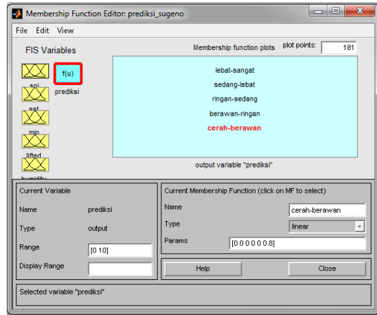
Gambar 12. MF output (prediksi) tipe Sugeno
