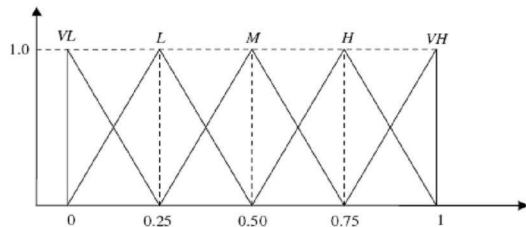
Gambar 0. Fungsi keanggotaan nilai-nilai linguistik untuk penilaian kriteria
