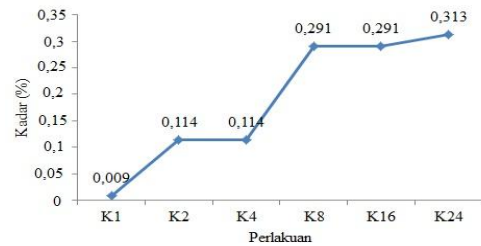
Gambar 13. Grafik Kadar Distribusi Total Asam glutamat pada Kolom Air Laut
