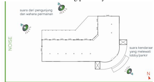
Gambar 5. Indexing sumber kebisingan
