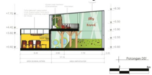
Gambar 16. Potongan D-D'
