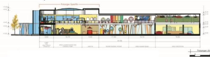
Gambar 13. Potongan A-A'
