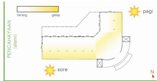
Gambar 4. Indexing pencahayaan alami
