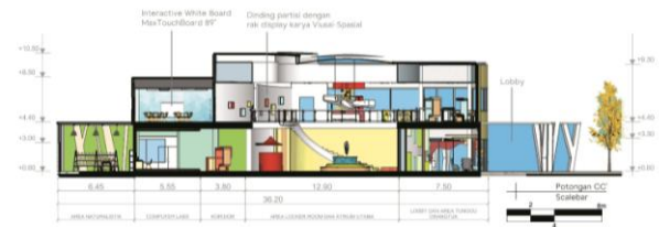
Gambar 15. Potongan C-C'
