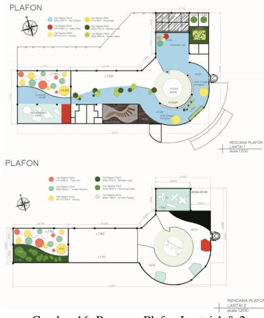
Gambar 16. Rencana Plafon Lantai 1 & 2
