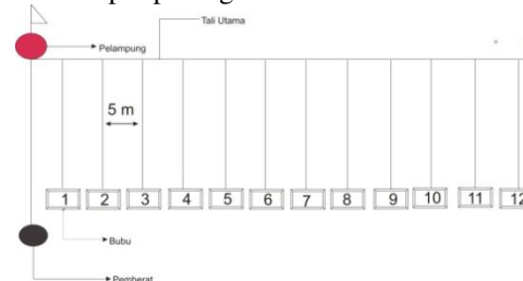
Gambar 1. Satu Rangkaian Bubu
