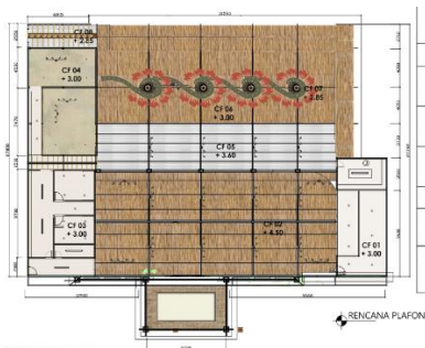
Gambar 14. Rencana Plafon
