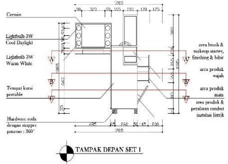
Gambar 12. Tampak Atas dan Depan Mebel 1
