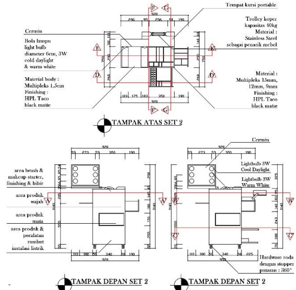
Gambar 16. Tampak Atas dan Depan Mebel 2
