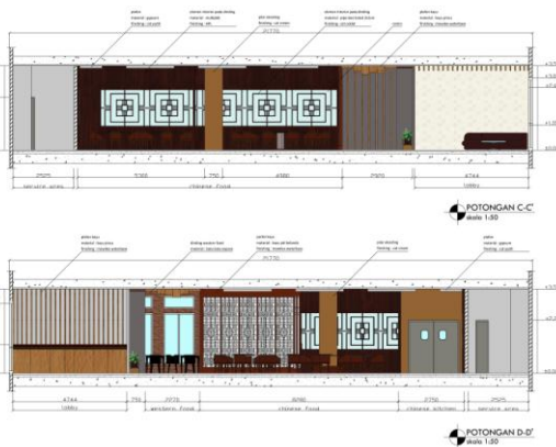
Gambar 7. Potongan C-C' dan Potongan D-D'
