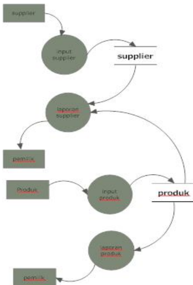
Gambar 5 Level 2 DFD
