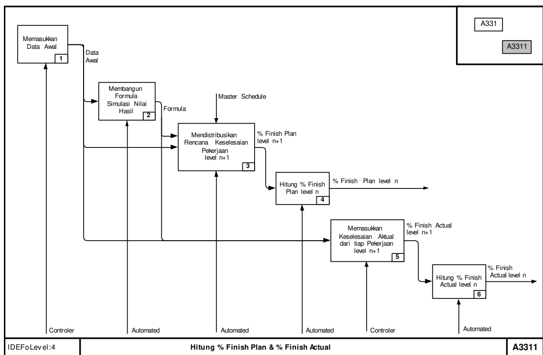
Gambar 5. IDEF0 Level 4 Hitung % Finish Plan & % Finish Actual
