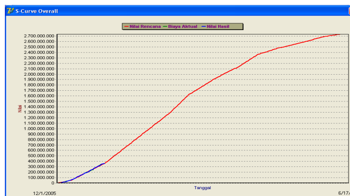
Gambar 16. Form Kurva-S
