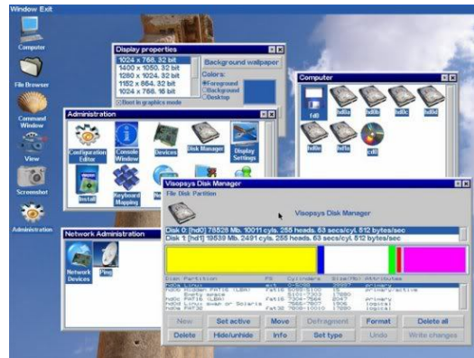
Gambar 8 Contoh Tampilan Visopsys
