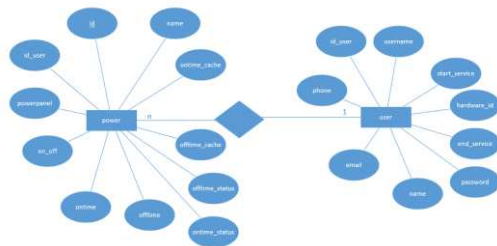
Gambar 6. ERD
