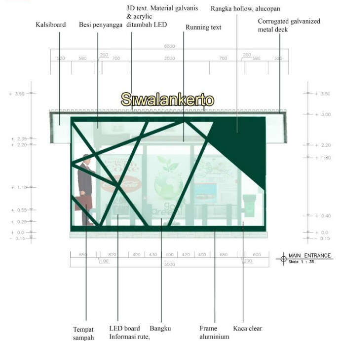
Gambar 6.38. Tampak main entrance alternatif 3 Sumber: Penulis (2015)
