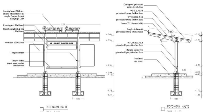
Gambar 7. Tampak potongan halte Sumber:Dinas Perhubungan Kota Surabaya (2014)
