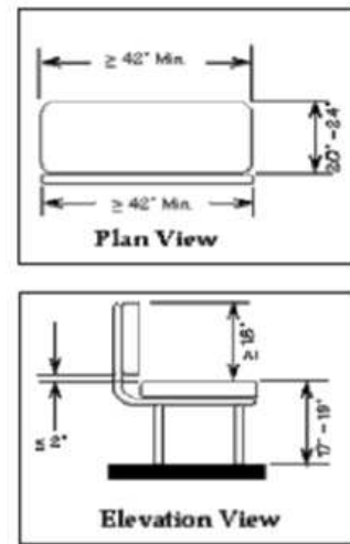
Gambar 3. Dimensi tempat duduk yang direkomendasikan Sumber: Guidelines for the Design and Placement of Transit Stops (2009, p.14)
