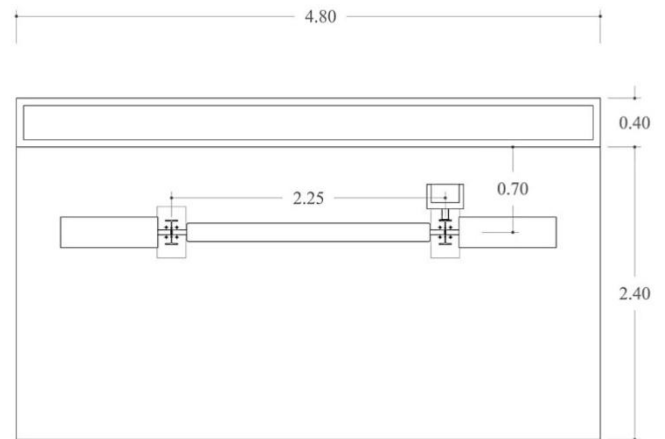
Gambar 6. Layout eksisting halte Sumber:Dinas Perhubungan Kota Surabaya (2014)
