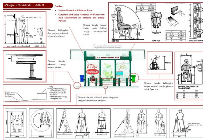
Gambar 6.40. Detail standards alternatif 3 Sumber: Penulis (2015)
