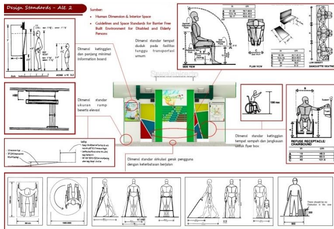
Gambar 6.35. Detail standards alternatif 2 Sumber: Penulis (2015)
