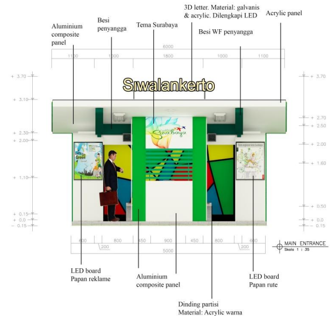
Gambar 6.33. Tampak main entrance alternatif 2 Sumber: Penulis (2015)
