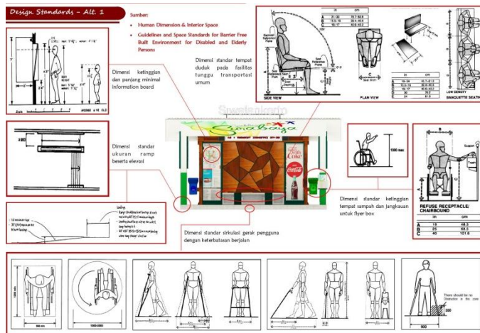
Gambar 6.30. Detail standards alternatif 1 Sumber: Penulis (2015)
