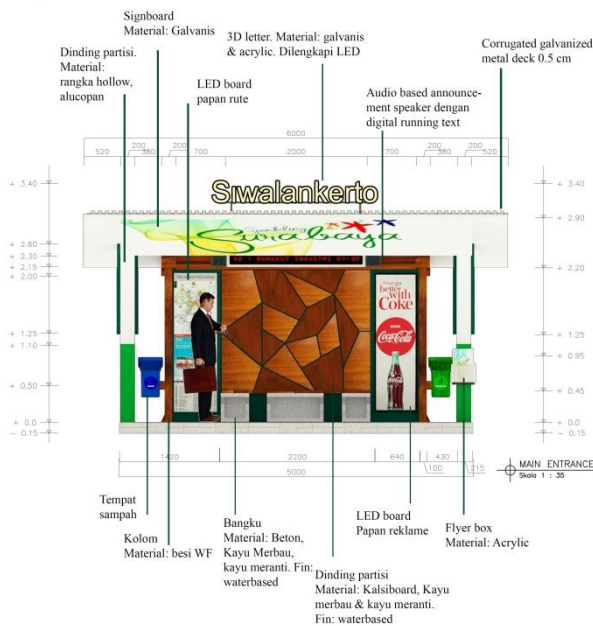
Gambar 6.28. Tampak main entrance alternatif 1 Sumber: Penulis (2015)
