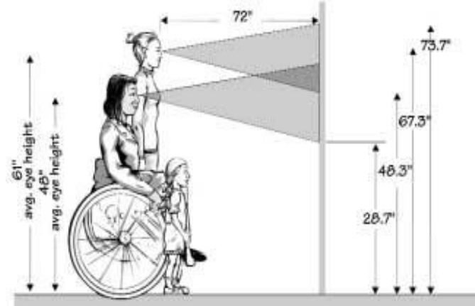
Gambar 2. Ketinggian papan informasi yang direkomendasikan Sumber: Guidelines for the Design and Placement of Transit Stops (2009, p.12)
