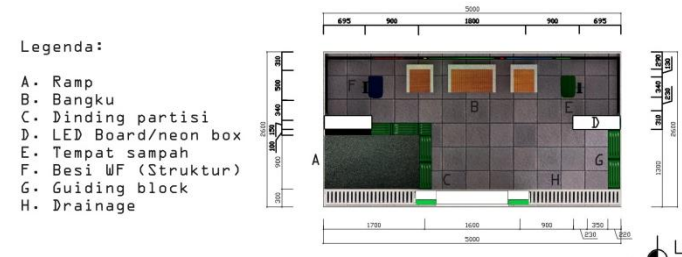
Gambar 6.32. Tampak layout alternatif 2 Sumber: Penulis (2015)
