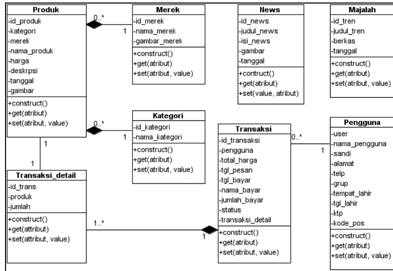
Gambar 3.3 Diagram Hubungan antar Entity Class .
