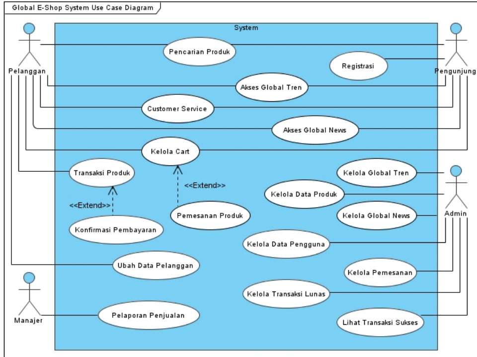
Gambar 3.1 System Use Case Diagram pada Global E-Shop
