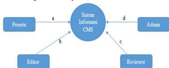
Gambar 2. Diagram Kontek Sistem Informasi CMS
