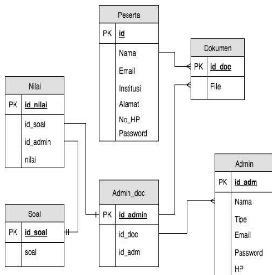
Gambar 5. Relasi Antar Tabel
