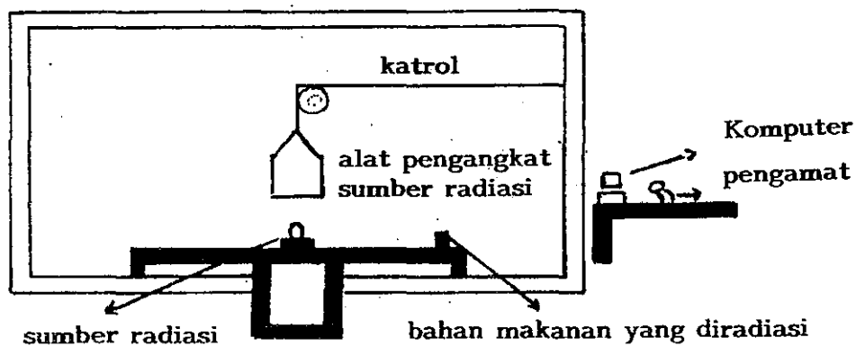
Gambar 2 Ruangan untuk meradiasi dan sumber radiasi saat digunakan untuk meradiasi
