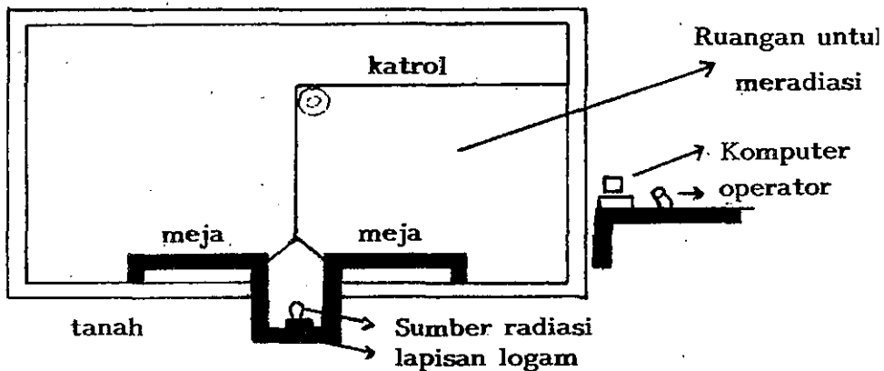
Gambar 2 Ruangan untuk meradiasi dan sumber radiasi saat digunakan untuk meradiasi
