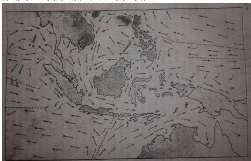
Gambar 23. pola arus Wyrтки bulan Februari (Wyrтки, 1961)
