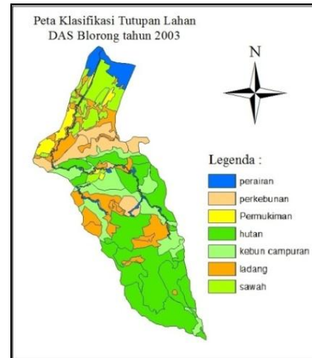
Gambar 3. Peta Klasifikasi Tutupan Lahan DAS Blorong tahun 2003
