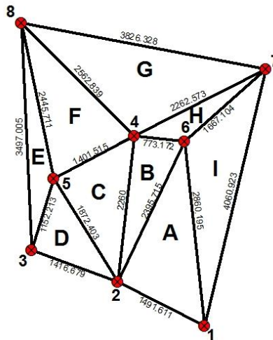
Gambar 7 Jaring segitiga GCP
