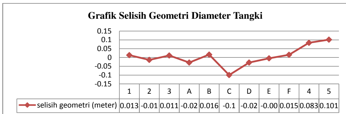
Gambar 12. Selisih geometri diameter tangki
