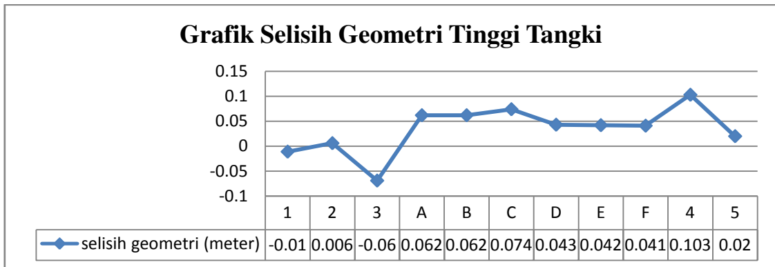
Gambar 11. Selisih geometri tinggi tangki
