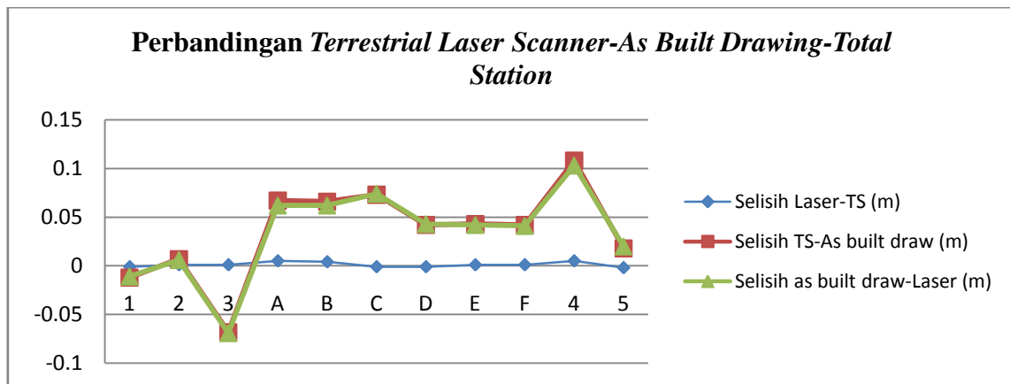
Gambar 13. Grafik perbandingan geometri tinggi tangki dengan Total Station Sokia Set 630R
