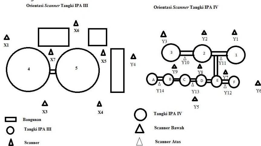
Gambar 4. Orientasi scanner tangki unit IPA III dan IPA IV
