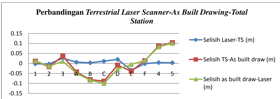
Gambar 14. Grafik perbandingan geometri tinggi tangki dengan Total Station Sokia Set 630R
