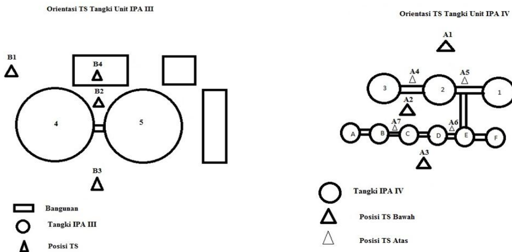
Gambar 8. Orientasi total station terhadap Tangki IPA III dan IPA IV
