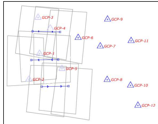
Gambar IV.3 Persebaran GCP pada Foto Udara 2 Basis
