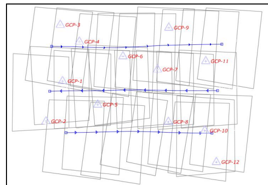
Gambar IV.1 Persebaran GCP pada Foto Udara 8 Basis
