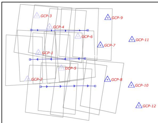
Gambar IV.2 Persebaran GCP pada Foto Udara 4 Basis
