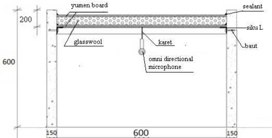
Gambar 2. Potongan Model Benda Uji dalam Ukuran Sebenarnya (ukuran dalam mm)
