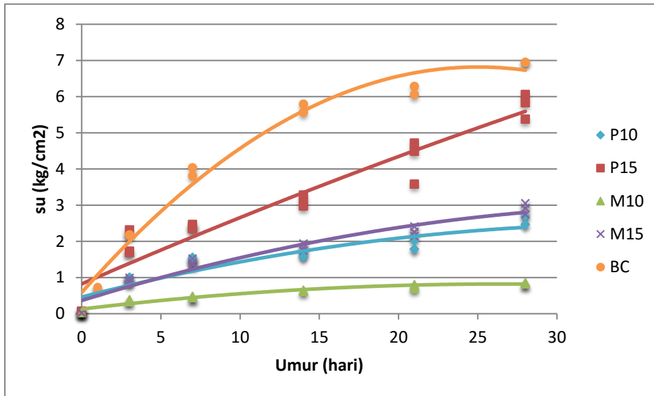
Gambar 1. Hasil Kuat Geser setiap Campuran Berbanding Umur
