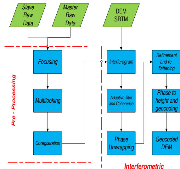
Gambar III.2. Tahapan Pengolahan ALOS PALSAR
