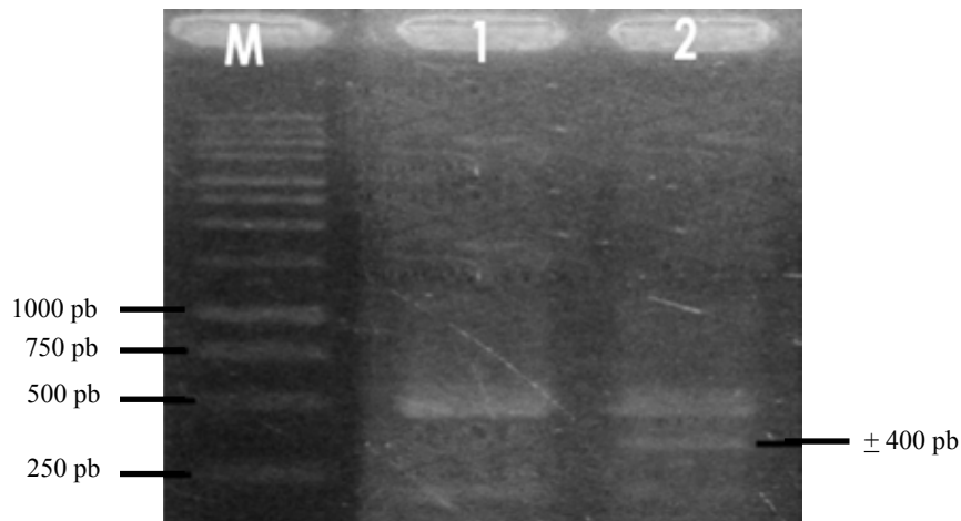
Gambar 2. Hasil elektroforesis dari amplifikasi DNA manggis. M = 1 kb, 1 = buah manggis bergetah kuning, 2 = buah manggis tidak bergetah kuning ( Electrophoresis result from DNA amplification on mangosteen. M = 1 kb, 1 = mangosteen with yellow latex, 2 = mangosteen without yellow latex )
