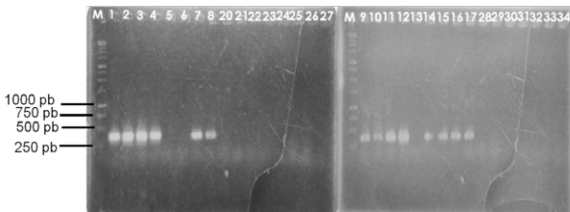
Gambar 3. Hasil elektroforesis dari amplifikasi DNA manggis. M = 1 kb; 1–17 aksesori manggis buah tidak bergetah dan 20–34 aksesori manggis bergetah kuning ( Electrophoresis result from DNA amplification on mangosteen. M = 1 kb; 1–17 mangoesteen accession without yellow latex; 20–34 mangoesteen accession with yellow latex )
