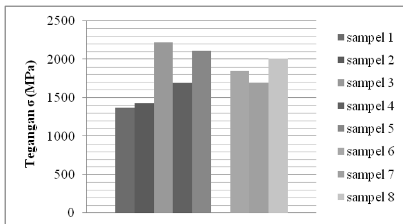
Gambar 5. Barchart Perbandingan Rangkaian Polyethylene Strap dengan Gabion
