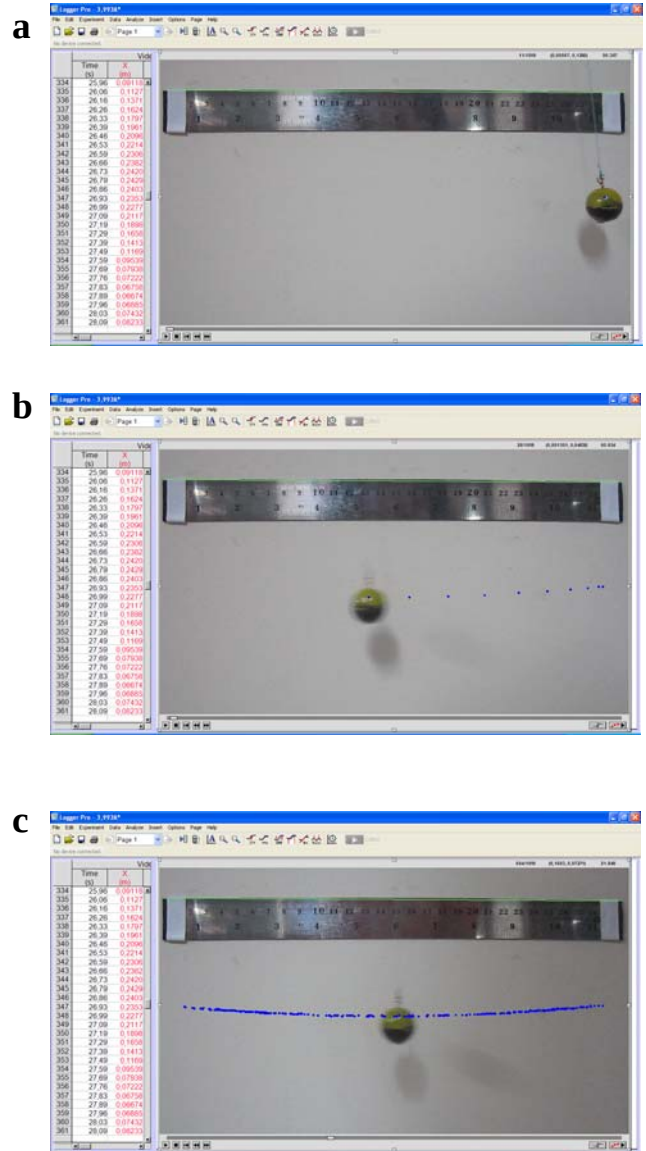
Gambar 2. Posisi setiap saat pada ayunan dengan beban bermassa 3,053 g dan panjang tali 120 cm. Ayunan diperlihatkan hanya pada bagian bebannya, tidak seluruhnya, agar memudahkan pelacakan kedudukan beban.
