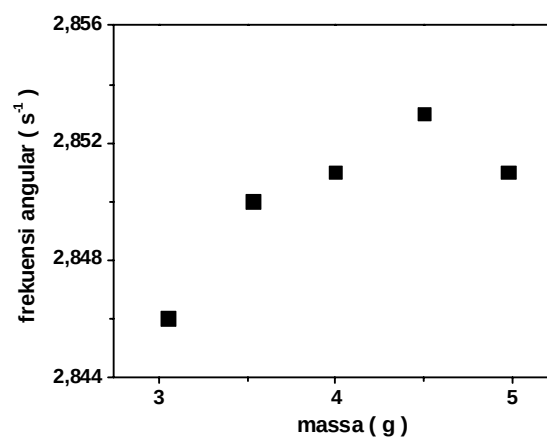
Gambar 5. Grafik hubungan antara frekuensi angular \omega ( \text{s}^{-1} ) dengan massa beban (g).
