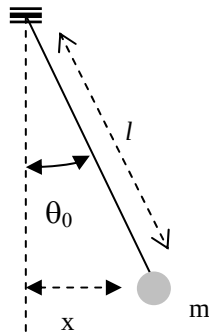
Gambar 1. Ayunan dengan panjang tali penggantung l , beban bermassa m disimpangkan dengan sudut awal \theta_0 dan simpangan horisontal sebesar x .
