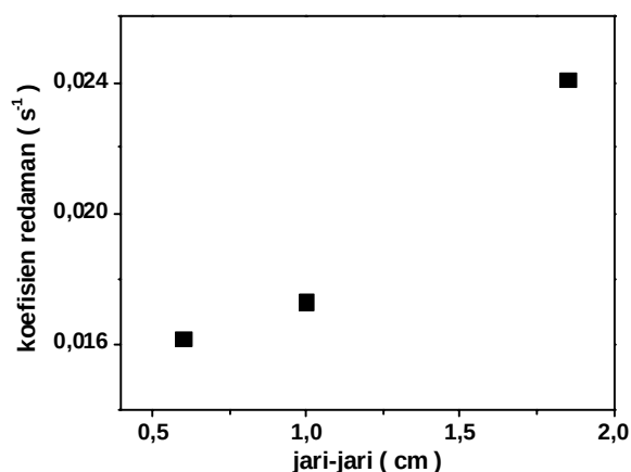
Gambar 6. Grafik hubungan antara koefisien redaman \beta ( \text{s}^{-1} ) dengan jari-jari beban (cm).
