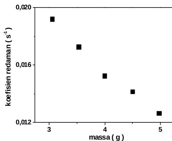
Gambar 4. Grafik hubungan antara koefisien redaman \beta ( \text{s}^{-1} ) dengan massa beban (g).
