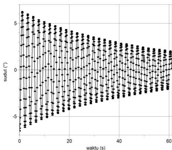
Gambar 3. Sudut simpangan fungsi waktu pada ayunan dengan beban bermassa 3,053 g, jari-jari beban 1 cm dan panjang tali 120 cm..
