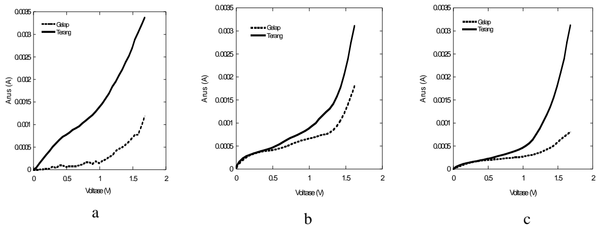
Gambar 1. Karakteristik I-V Elkahfi (a) elektrolit KI, (b) elektrolit NaI, dan (c) elektrolit TEAI
