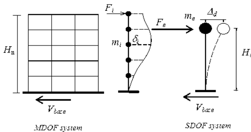
Gambar 2. Permodelan SDOF dari Bangunan Bertingkat
