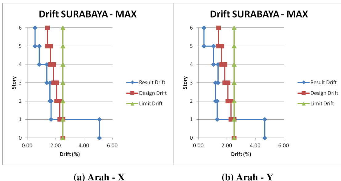
Gambar 3. Grafik Perbandingan Hasil Drift Ratio Bangunan Surabaya
