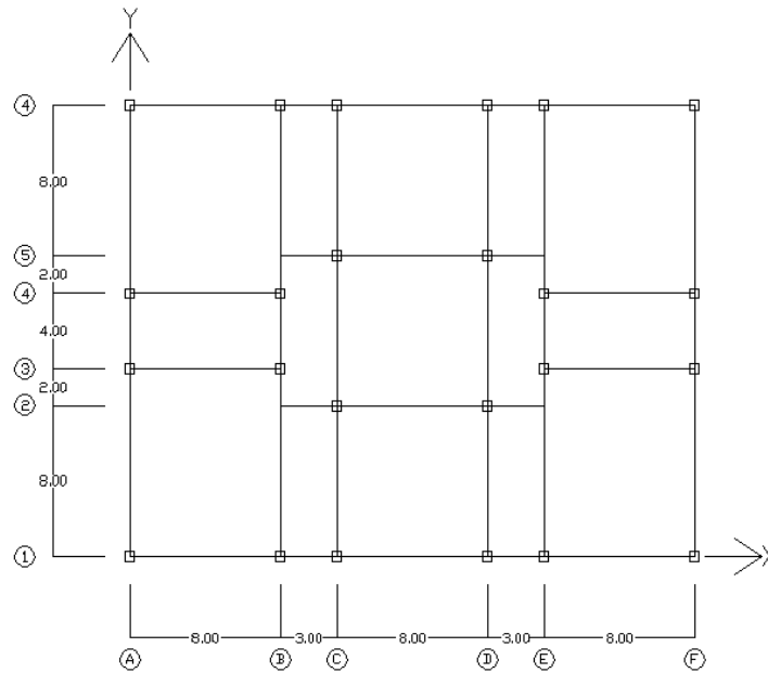
Gambar 1. Denah Struktur Bangunan
