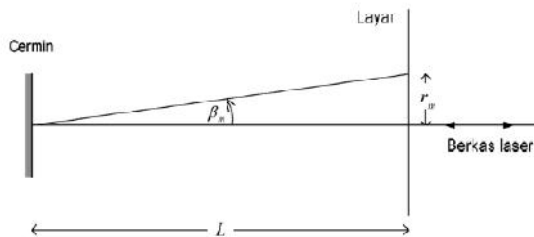
Gambar 1. Koordinat sudut \beta_m dan jejari cincinterang r_m , serta jarak layar-cermin L
