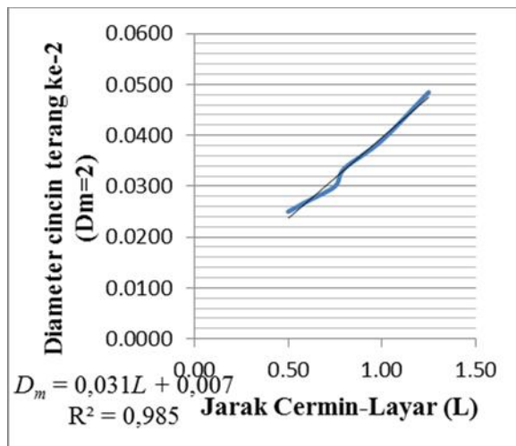
Gambar 5. Grafik D_m versus L untuk m = 2 pada Laser He-Ne. Garis lurus adalah hasil analisis regresi linear menggunakan MS Excel dan memiliki persamaan D_{m=1} = 0,021L + 0,006 (dalam meter).
