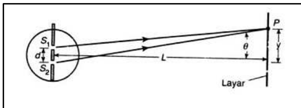
Gambar 1. Konfigurasi interferensi celah 2 Young (Sugito et al. 2005)
