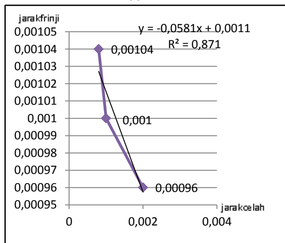
Gambar 5. Grafik pengaruh jarak antar celah ( d ) terhadap jarak frinji ( y ) pada Laser He-Ne menggunakan celah 5
