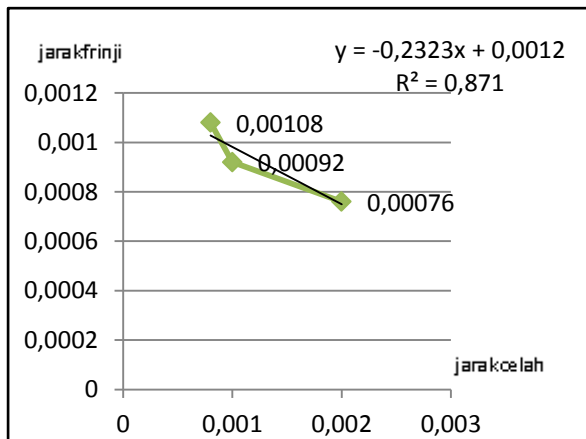
Gambar 5. Grafik pengaruh jarak antar celah ( d ) terhadap jarak frinji ( y ) pada Laser He-Ne menggunakan celah 5
