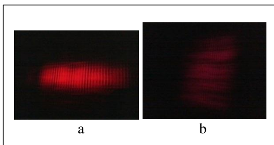
Gambar 6. Pola interferensi celah 5 (a) laser He-Ne dan (b) laser dioda ( d=0,00092 m; L=2,5 m)
