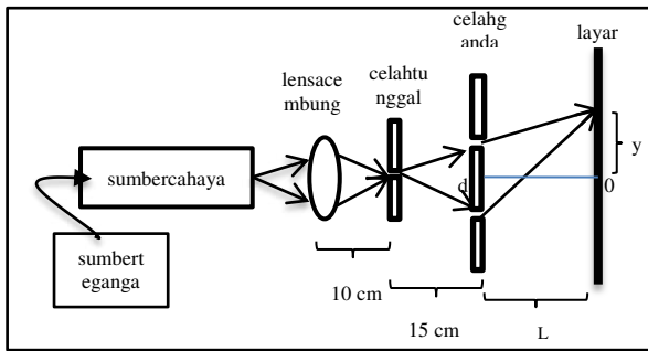
Gambar 2. Rangkaian alat eksperimen
