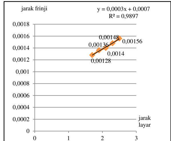
Gambar 3. Grafik pengaruh jarak layar (L) dan jarak frinji (y) pada Laser He-Ne menggunakan celah 5
