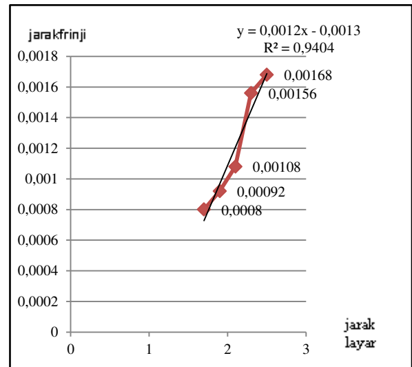
Gambar 4. Grafik pengaruh jarak layar (L) dan jarak frinji (y) pada Laser dioda menggunakan celah 5
