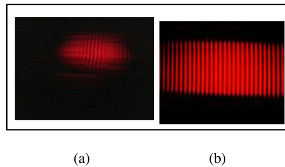
Gambar 7. Pola interferensi laser He-Ne (a) penelitian ini (b) Sugito et al. (2005)
