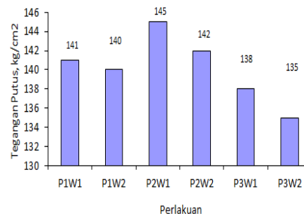
Gambar 2. Tegangan putus ( \text{kg/cm}^2 ) kompon ban dalam kendaraan bermotor roda dua
