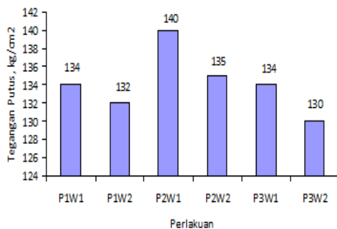
Gambar 5. Perubahan Tegangan Putus ( \text{kg/cm}^2 ) Kompon Ban dalam Kendaraan Bermotor
