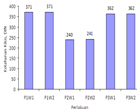
Gambar 3. Ketahanan kikis (DIN, mm) kompon ban dalam kendaraan bermotor
