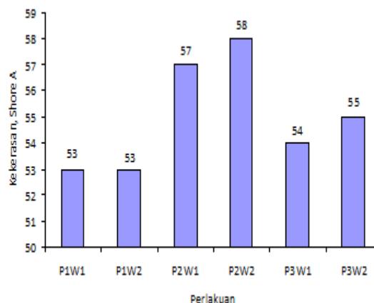
Gambar 4. Perubahan kekerasan ( Shore A ) kompon ban dalam kendaraan bermotor roda dua setelah pengusangan
