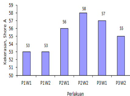
Gambar 1. Kekerasan ( Shore A ) kompon ban dalam kendaraan bermotor roda dua
