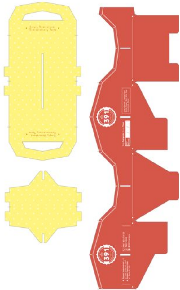
Gambar 28. Pola Jejaring Kemasan Sekunder Pie in Jar (tray)
