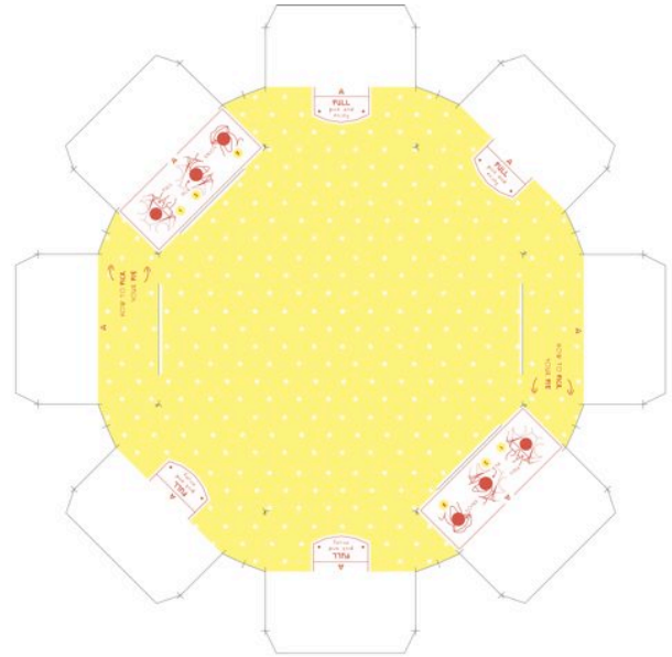
Gambar 24. Pola Jejaring Kemasan Primer 9 Mini Pie (alas)
