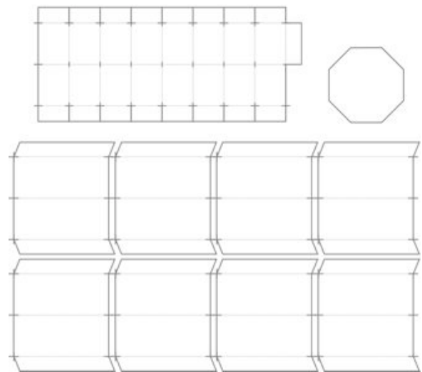
Gambar 25. Pola Jejaring Kemasan Primer 9 Mini Pie (sekat)
