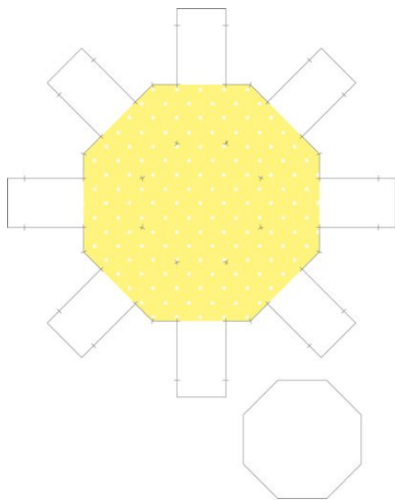
Gambar 22. Pola Jejaring Kemasan Primer 1 Mini Pie (alas)
