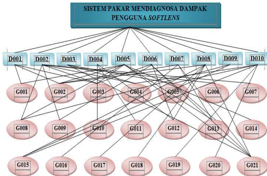
Gambar 7. Pohon Keputusan
