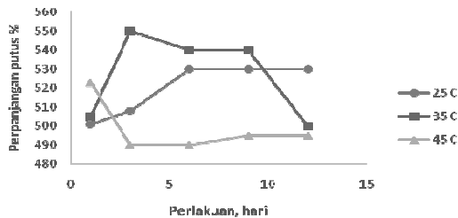
Gambar 9. Perpanjangan putus kompon karet lis kaca kendaraan bermotor selama penyimpanan (90 phr silika)
