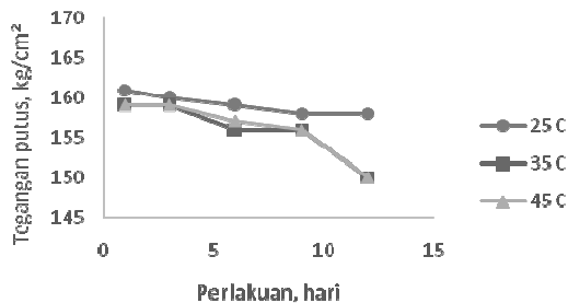
Gambar 7. Tegangan putus kompon karet lis kaca kendaraan bermotor selama penyimpanan (90 phr silika)
