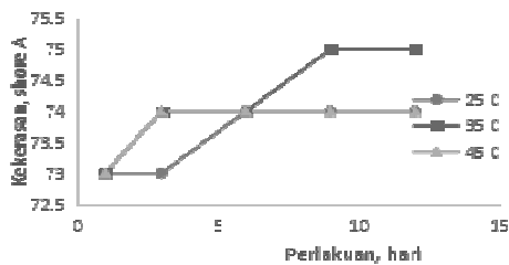
Gambar 5. Kekerasan kompon karet lis kaca kendaraan bermotor selama penyimpanan (90 phr silika).
