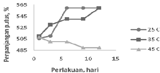
Gambar 8. Perpanjangan putus kompon karet lis kaca kendaraan bermotor selama penyimpanan (80 phr silika)
