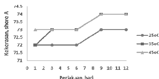
Gambar 4. Kekerasan kompon karet lis kaca kendaraan bermotor selama penyimpanan (80 phr silika)
