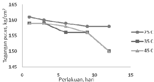
Gambar 6. Tegangan putus kompon karet lis kaca kendaraan bermotor selama penyimpanan (80 phr silika)
