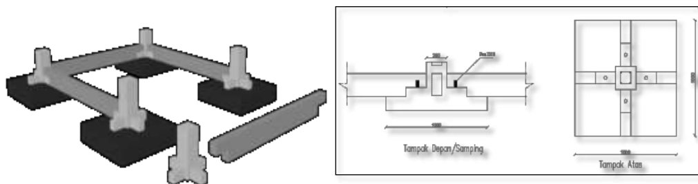
Gambar 3 Sistem Interlocking Tipe 4
