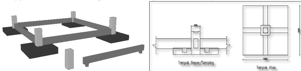
Gambar 2 Sistem Interlocking Tipe 3
