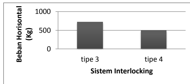
Grafik 1. Perbandingan Kemampuan Menahan Beban Horisontal
