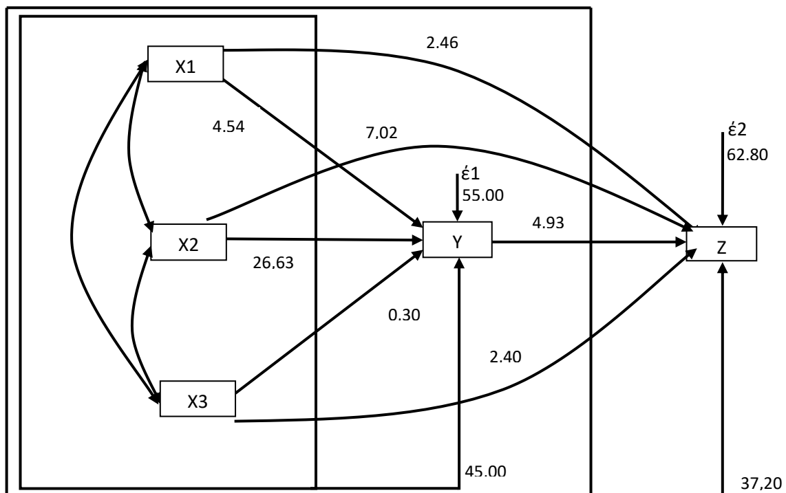
Gambar 2. Struktur Lengkap Diagram Jalur Hasil Pengujian Hipotesis Hubungan Kausal Antara variabel
